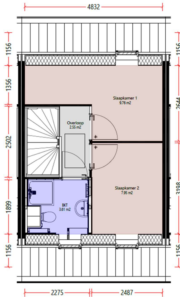
Verdieping_1e
